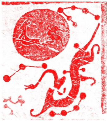
河南南阳出土的“东方苍龙”星座汉代画像石。
