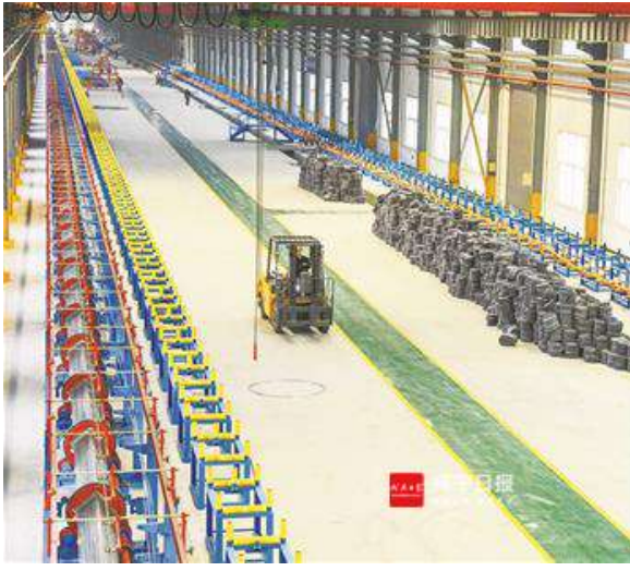
湖北欧特特绳索制品有限公司车间,这里生产的绳索特用于建设嘉鱼长江大桥。
